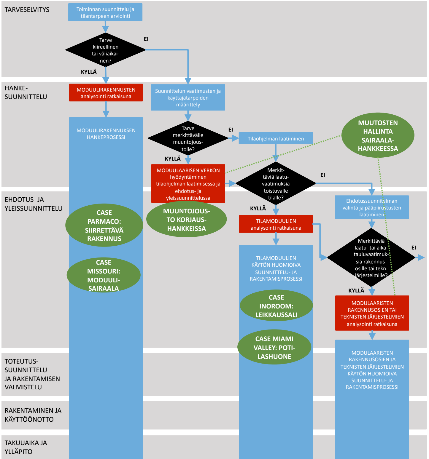
Kuva 1. Modulaarisuutta hyödyntävä rakennushankkeen prosessi. Vihreät pallot kuvaavat hankkeen osatutkimusten sijoittumista prosessiin.
