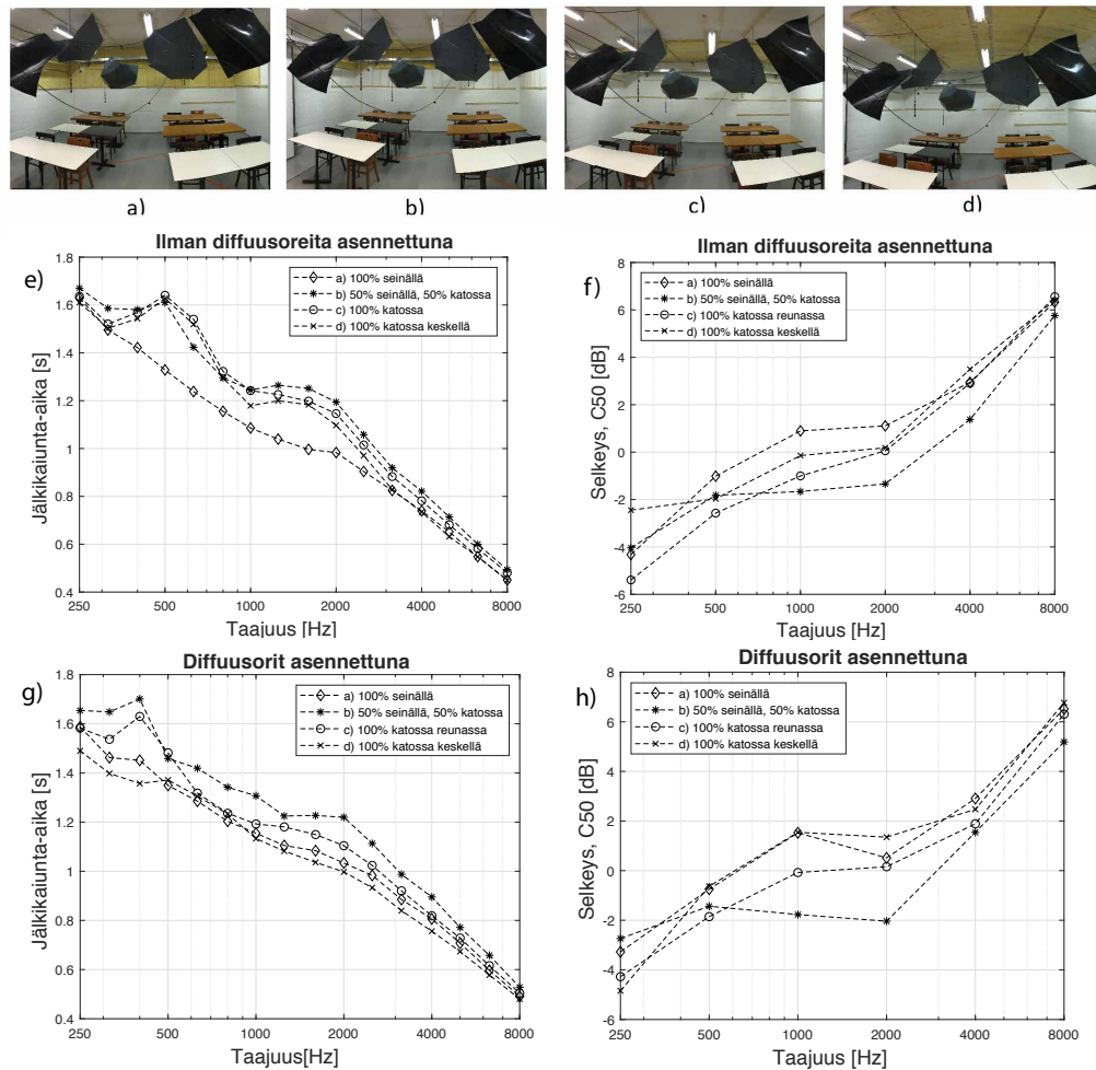
Kuva 2: Luokahuoneessa mitatut T_{20} ja C_{50} , vaimennusmateriaalina oli 50 mm lasivillaa asennettuna a) katon rajaan seinälle, b) puolet seinälle ja puolet kattoon, c) kattoon seinän vierustalle ja d) katon keskelle. Kuvissa e-f) on mittaustulokset ilman roikkuvia diffusoreita ja g-h) diffusoreiden kanssa.
