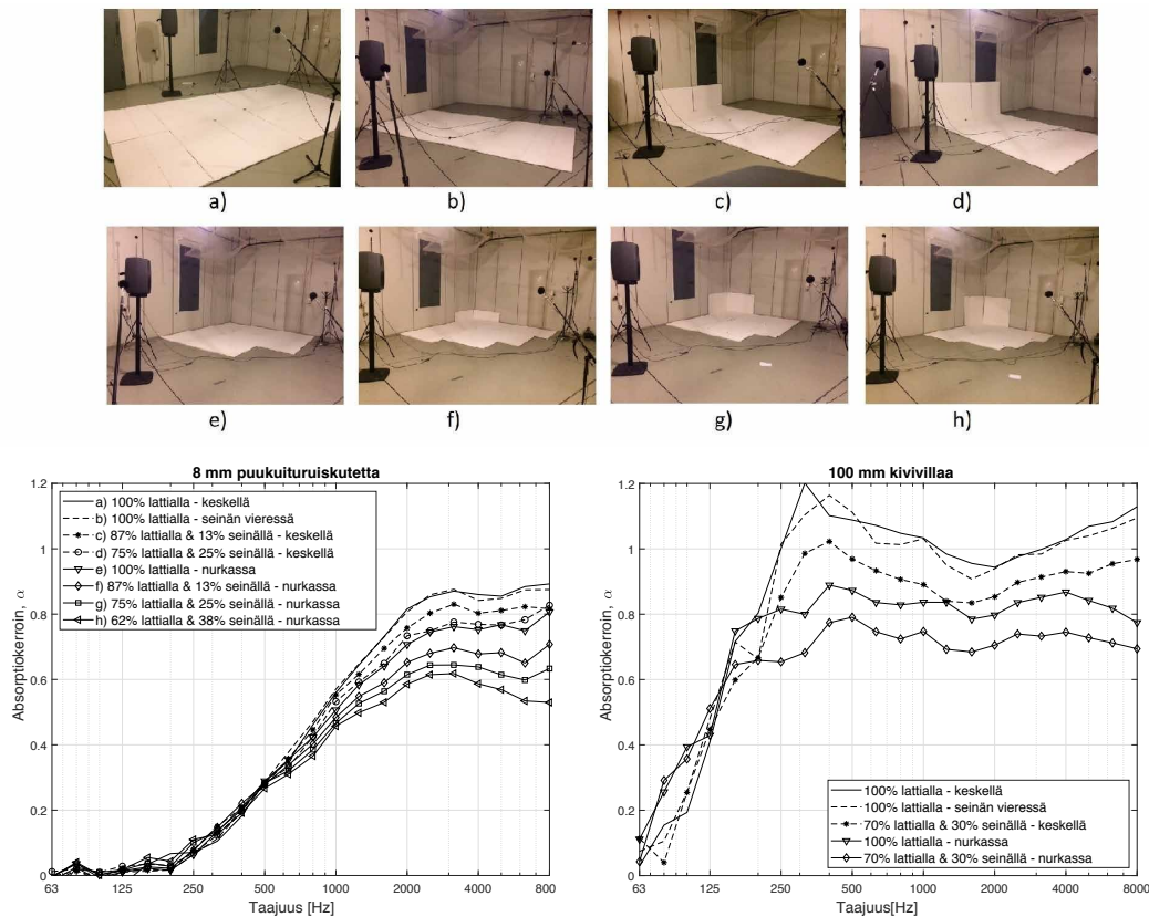
Kuva 1: Absorptiokertoimet: 8 mm ruiskutettua puukuitua (vasemmalla) ja 100 mm kivivillaa (oikealla) materiaalien ollessa a) huoneen keskellä, b) lähellä seinää, c-d) osoittain seinällä sekä e-h) huoneen nurkassa erilaisilla sijoitteluilla. Kuvissa on ruiskutetut puukuitulevyt.
