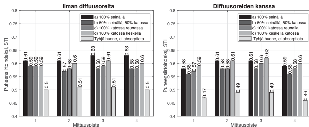
Kuva 3: Luokahuoneessa mitatut puheensiirtoindeksin arvot neljässä eri mittauspisteessä erilaisilla vaimennusmateriaalin sijoitteluilla sekä diffusoreiden kanssa että ilman.
