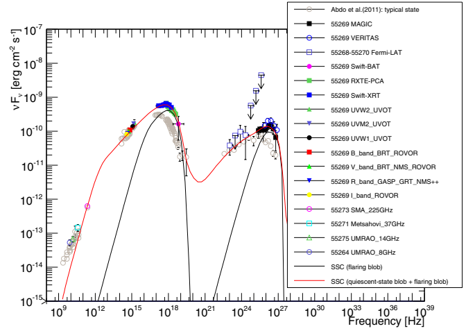
(d) MJD 55 269.
