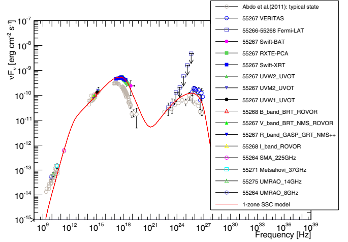
(b) MJD 55 267.
