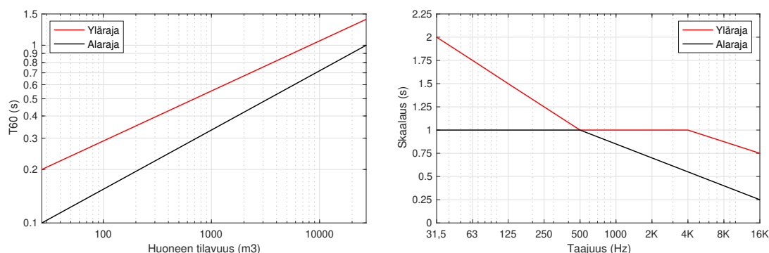
Kuva 1. Vasemmalla suositus elokuvateatterien ja miksaamojen jälkikaiunta-ajalle 500 Hz:n taajuudella huoneen tilavuuden mukaan. Oikealla jälkikaiunta-ajan pituuden vaihteluväli eri taajuuksilla.
