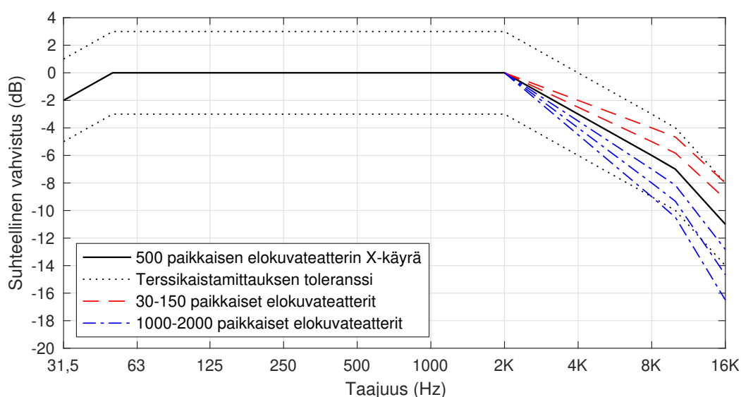
Kuva 2. 500 paikkaisen elokuvateatterin X-käyrä sekä sovitukset pienemmille ja suuremmille teattereille standardin SMPTE 202:2010 mukaisesti [11].
